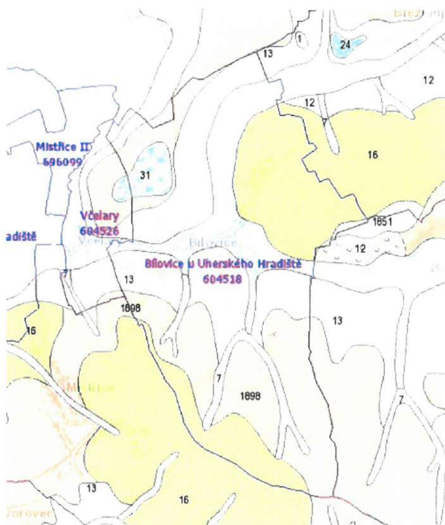
Obr. 1. Výřez z geologické mapy 1 : 50 000, k. ú. Bilovice u Uherského Hradiště. Legenda: 13 – hlinitojílovité až hlinitokamenité svahové sedimenty; 16 – spraše a sprašové hlíny; 31 – písky a štěrky, říční terasa; 1898 – flyšové střídání pískovců a jílovců (zdroj: www.geology.cz ).
